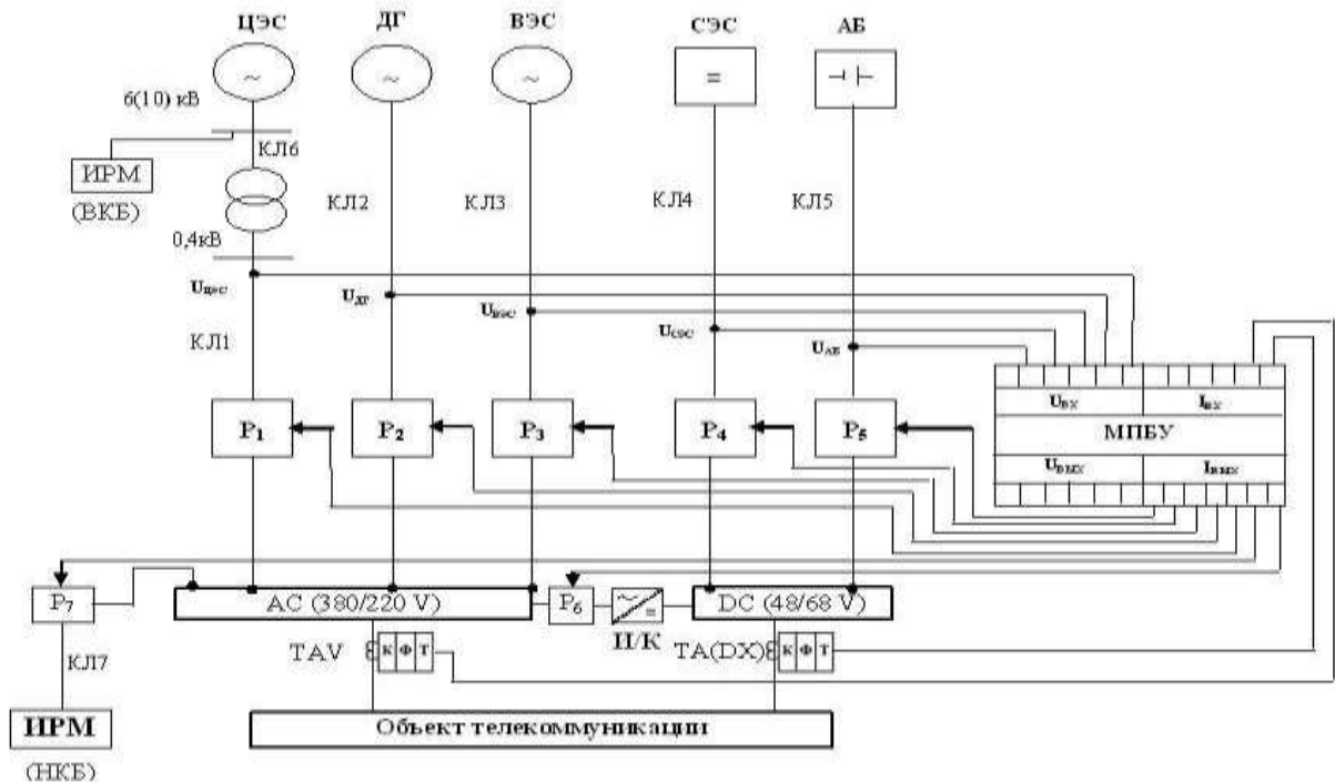
Рис.1. Схема соединения микропроцессорного блока комбинированного управления источниками реактивной мощности объекта телекоммуникации
